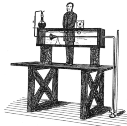
Figure : Expérience de Reynolds, O. Reynolds 1883, Domaine Public
