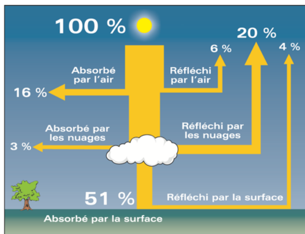
Figure : Bilan radiatif. S. Malardel 2009, Fondamentaux de Météorologie, Cépaduès.
